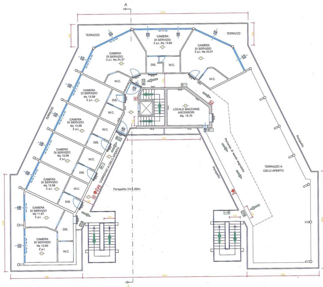
PIANTA PIANO SETTIMO
