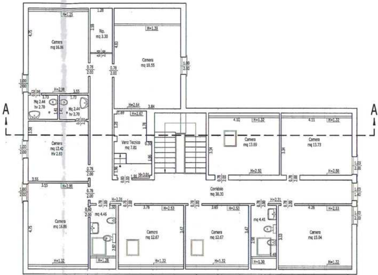
Piano Sottotetto
