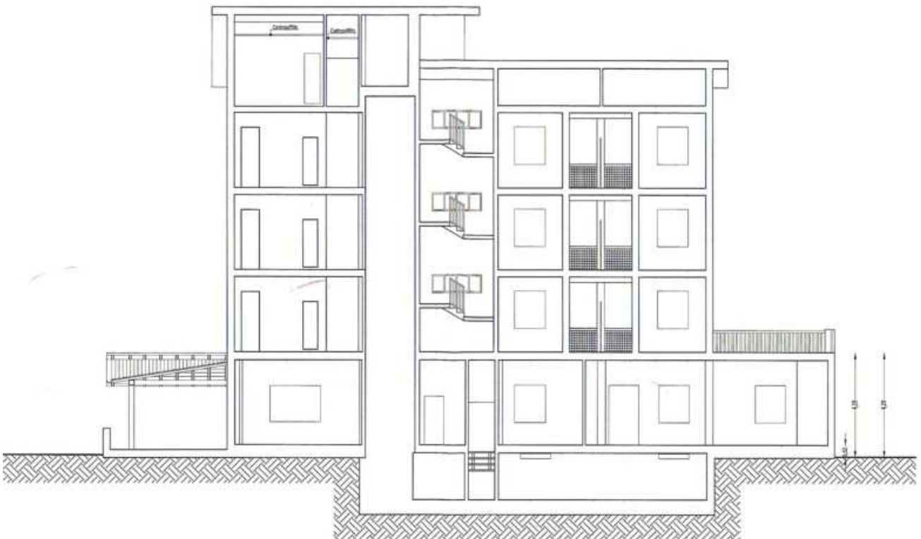
Sezione A:A
