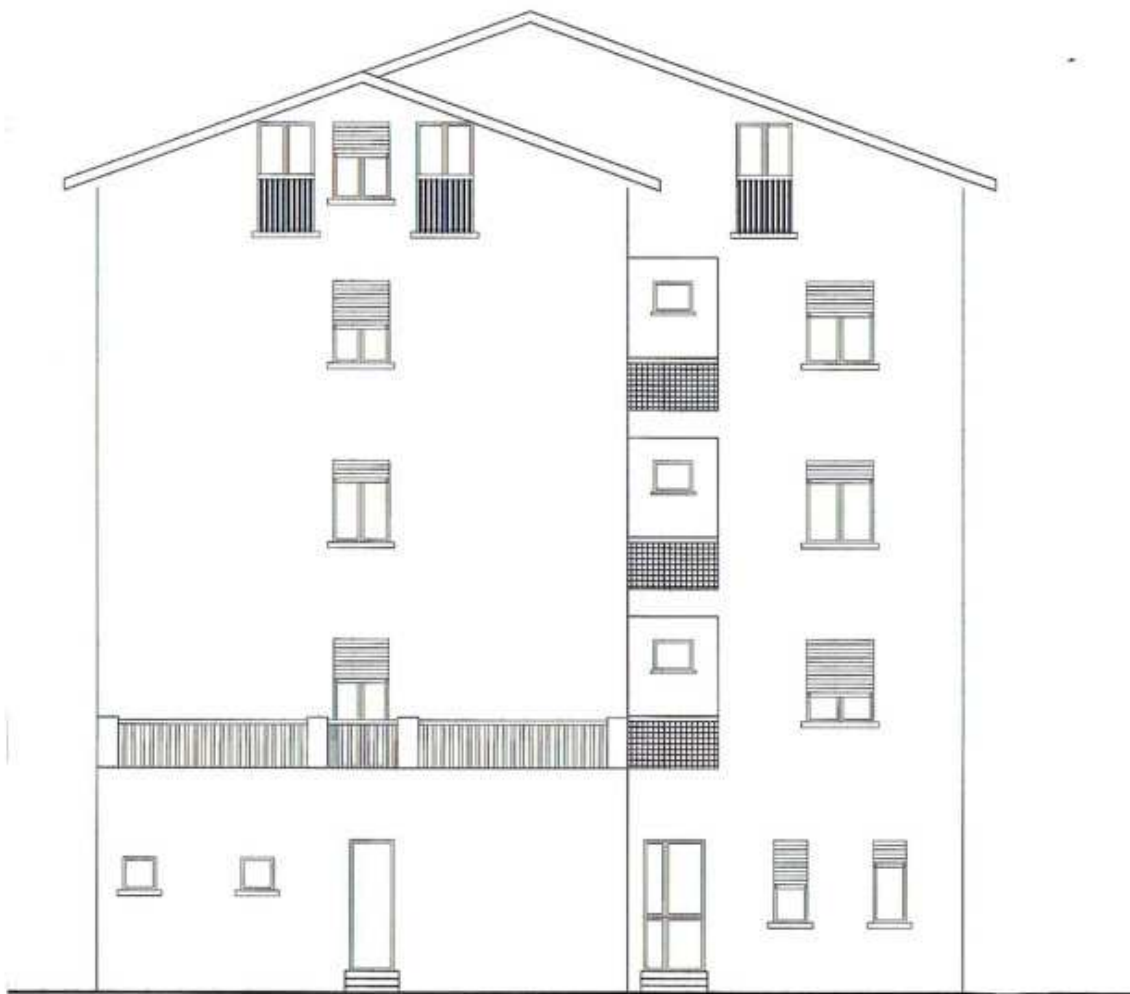
Prospetto lato Ravenna
