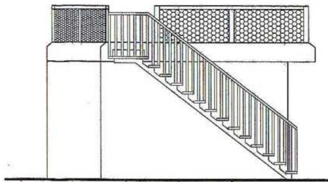
Prospetto Lato Sinistro
